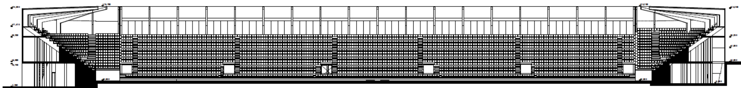
ŘEZ A-A
