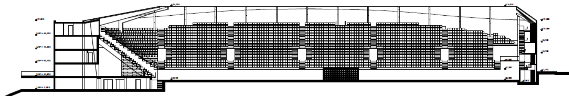
ŘEZ B-B
