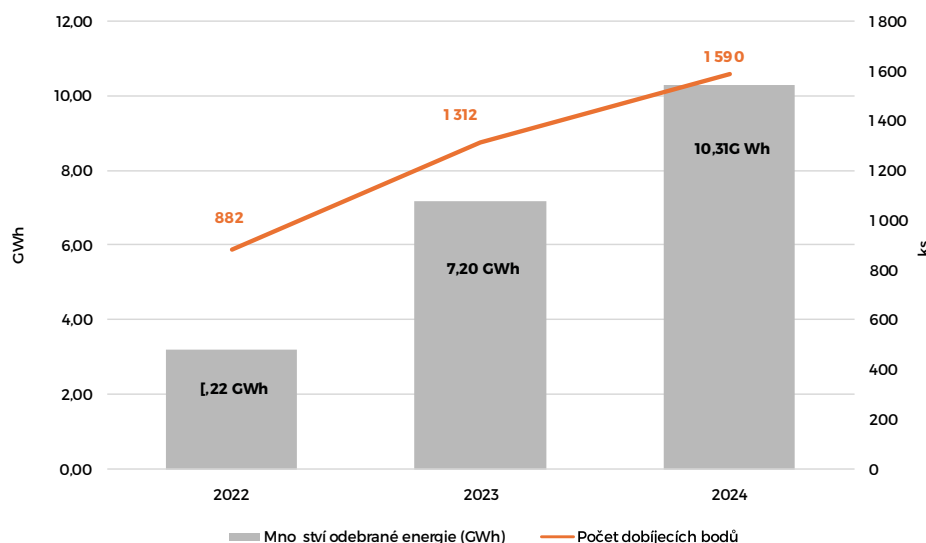
GRAF 10: Množství elektřiny odebrané z veřejných nabíjecích stanic a počet dobíjecích bodů (2022–2024)
